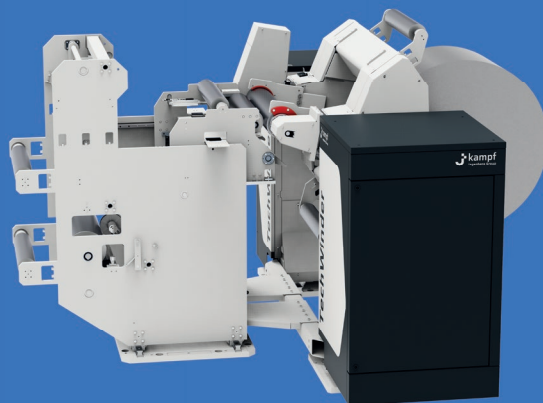
Wendeaufwickler
